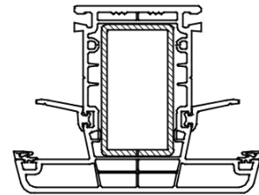
6054 tussenstijl
