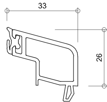
6130 glasdikte 29+30mm
