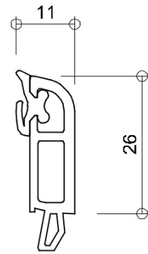
6152 glasdikte 51+52mm
