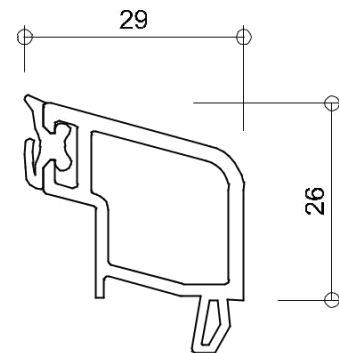
6134 glasdikte 33+34mm
