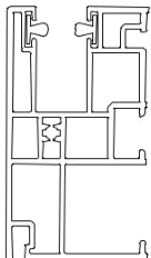
horizontale doorsnede geleidsprofiel rolluik
