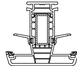
6050 tussenstijl
