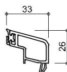
6130 glasdikte 30+31mm
